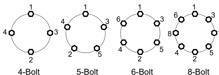
Wheel Lug Torque Pattern
