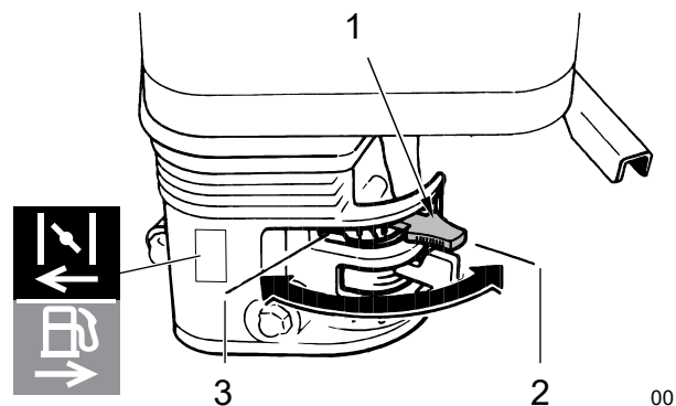
Fig. 6 —Manette d'étrangleur
