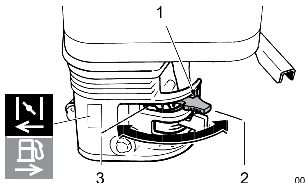
Fig. 19 – Manette d'étrangleur
